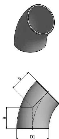
Curva 45°
