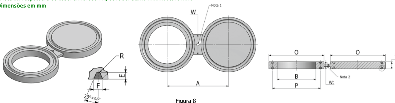
Figura 8 Face RTJ
