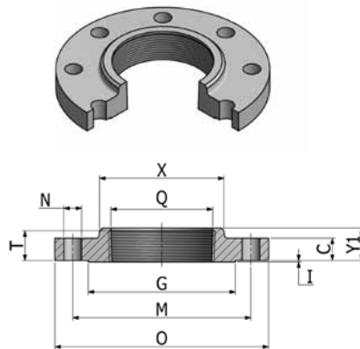
Flange Roscado
