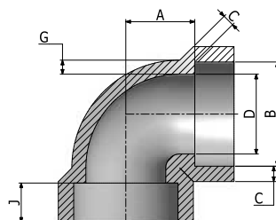
Cotovelo 90°
