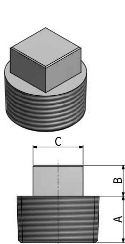
Plug Cabeça Quadrada
