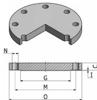
Flange Cego
