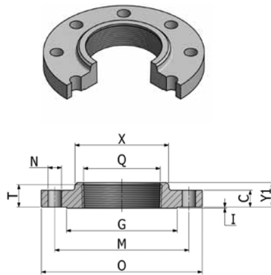
Flange Roscado
