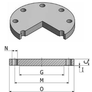
Flange Cego
