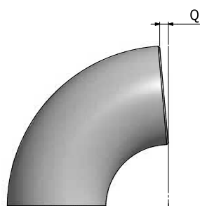
Curva
