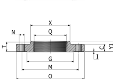
Flange Roscado
