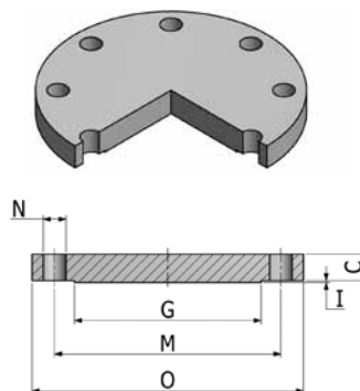
Flange Cego
