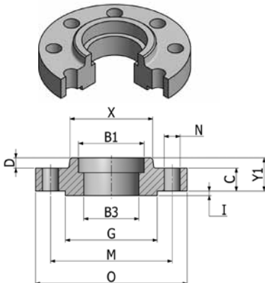
Flange Encaixe
