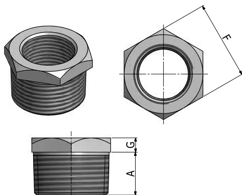
Bucha de Redução Sextavada
