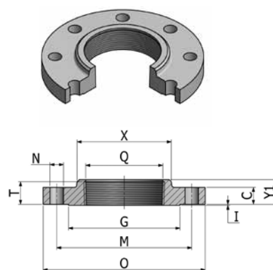
Flange Roscado
