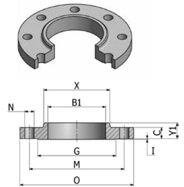
Flange Sobreposto
