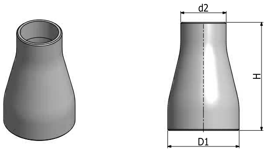
Redução Concêntrica
