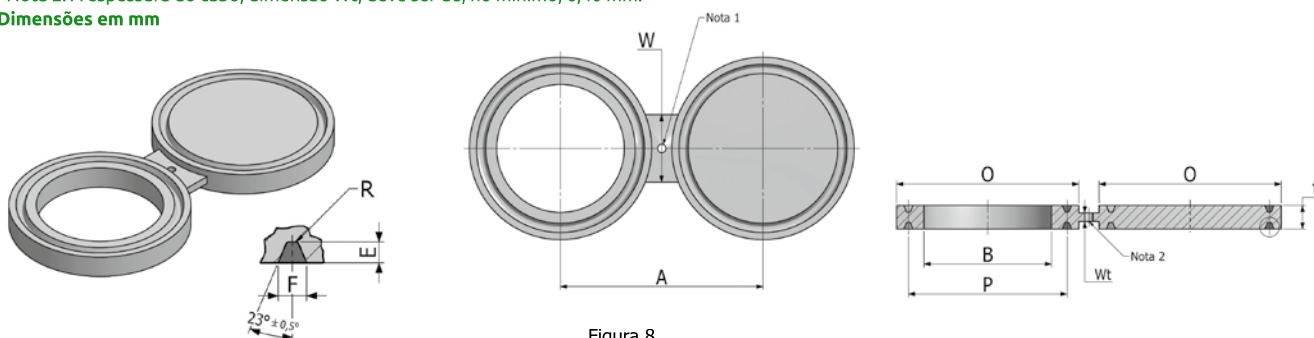
Figura 8 Face RTJ
