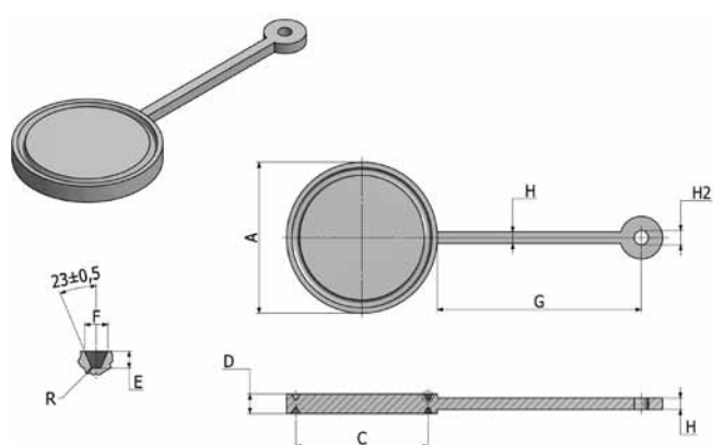
Raquete N120 C
