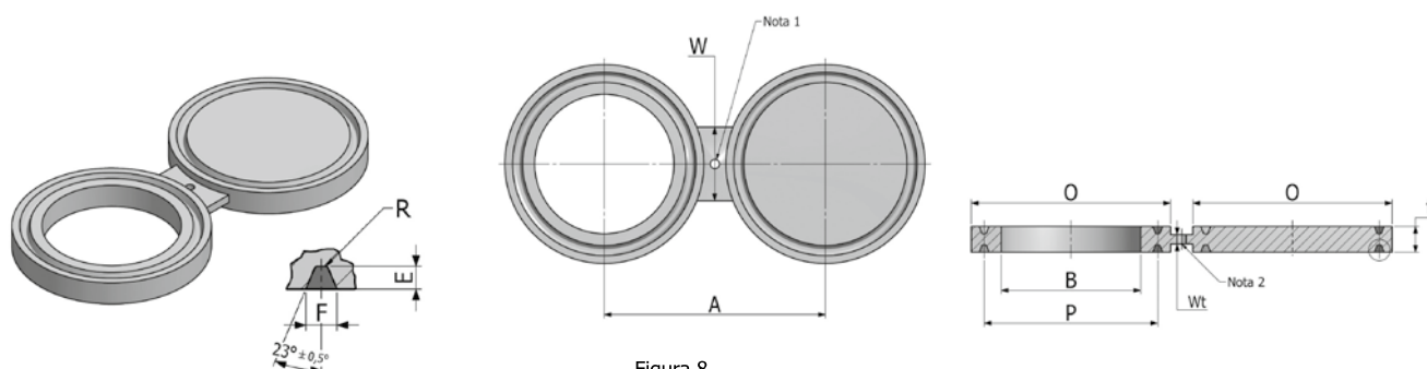
Figura 8 Canal RTJ
