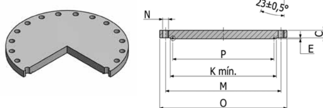
Flange Cego com Canal RTJ
