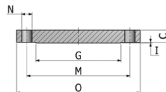
Flange Cego
