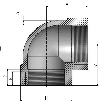
Cotovelo 90°
