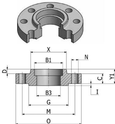
Flange Encaixe
