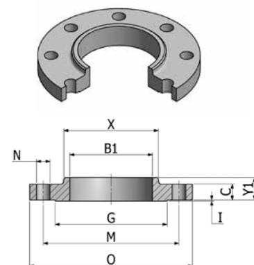
Flange Sobreposto
