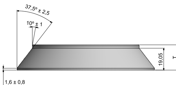
Redução
