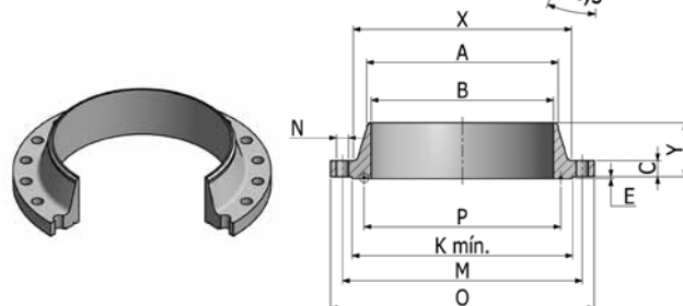
Flange FWN com Canal RTJ
