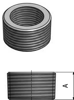
Bucha de Redução
