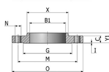
Flange Sobreposto
