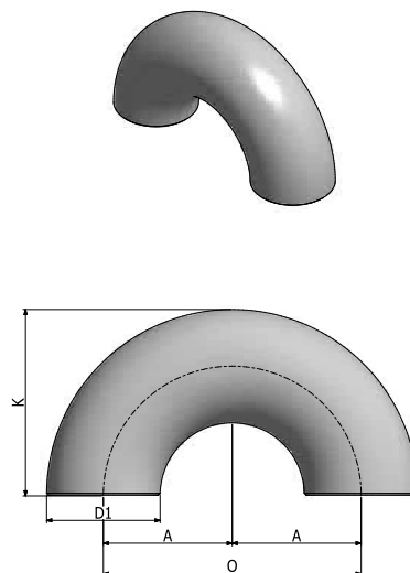
Curva 180°
