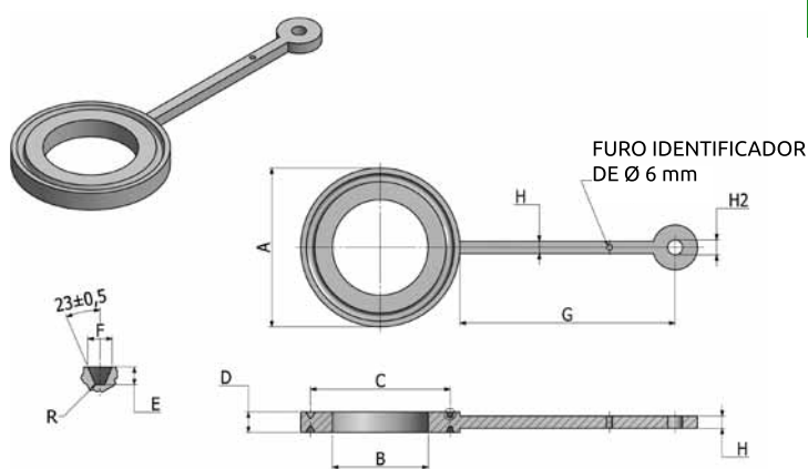
Anel Espaçador N120 C
